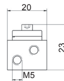
Tobera pulverizadora
